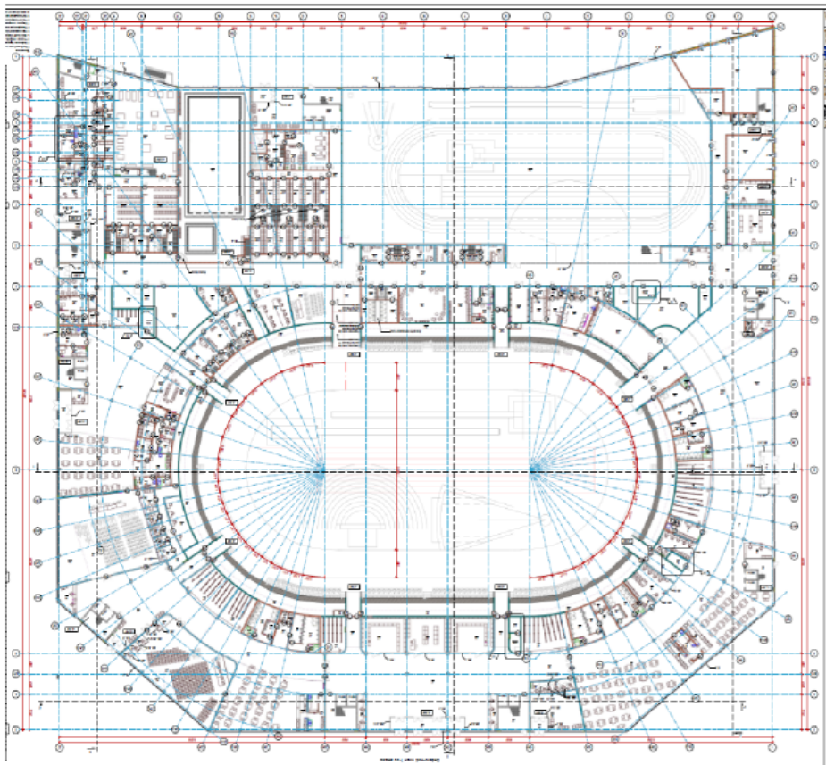
ПЛАН ЛЕГКОАТЛЕТИЧЕСКОГО СПОРТИВНОГО КОМПЛЕКСА
